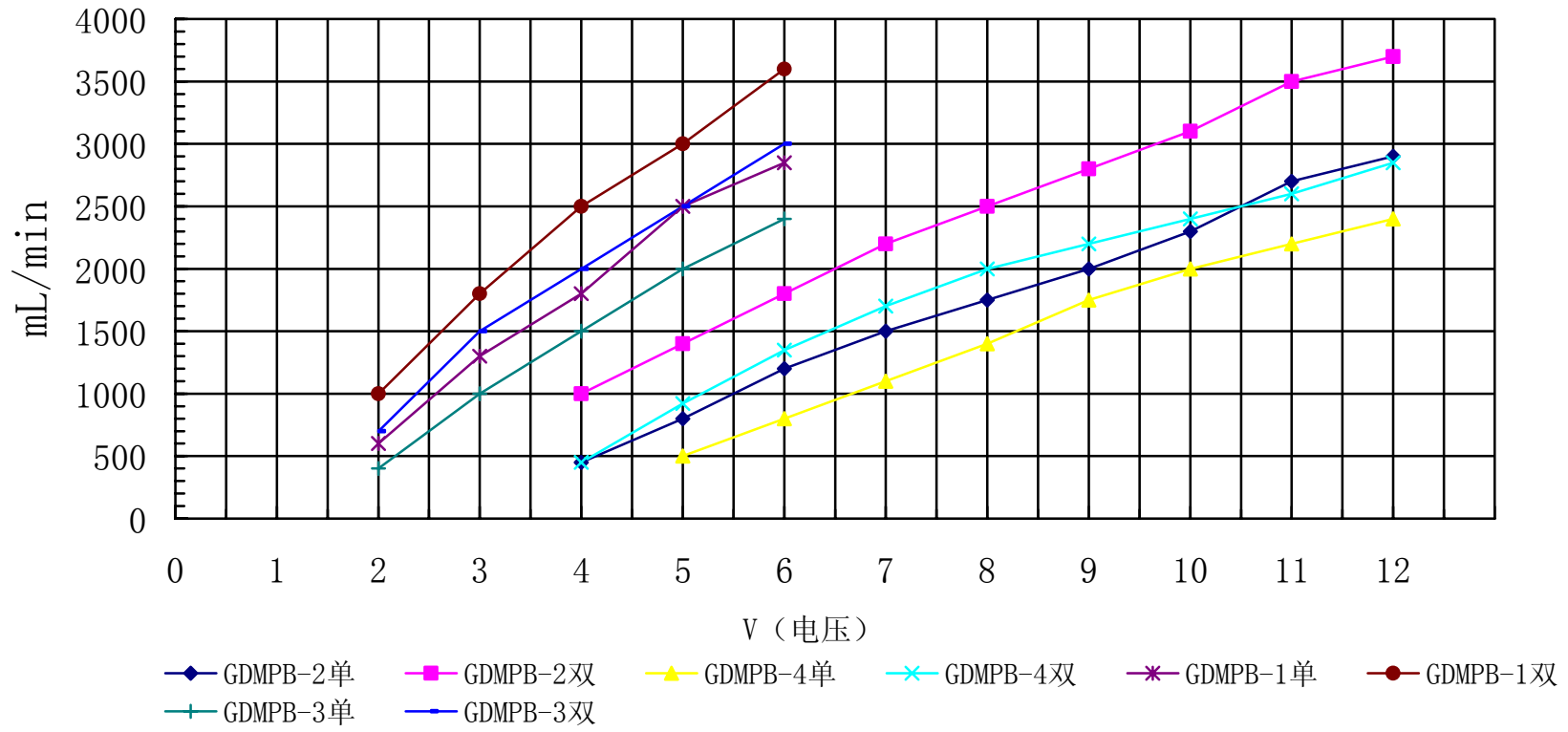
GDMPB电压流量图
