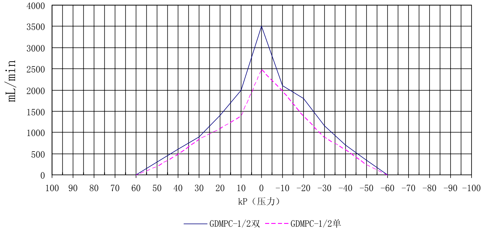
GDMPC系列流量负载图
