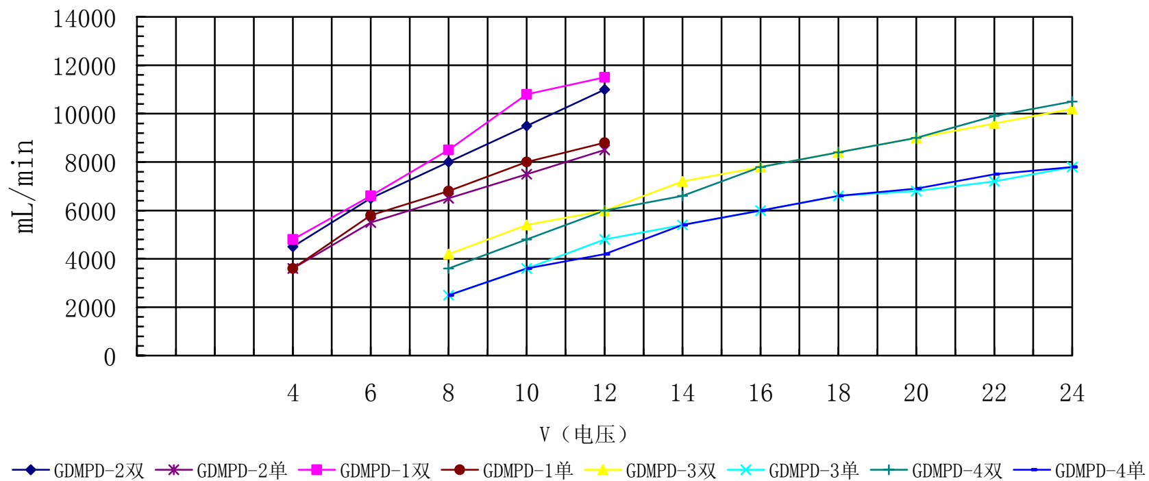
GDMPD电压流量图
