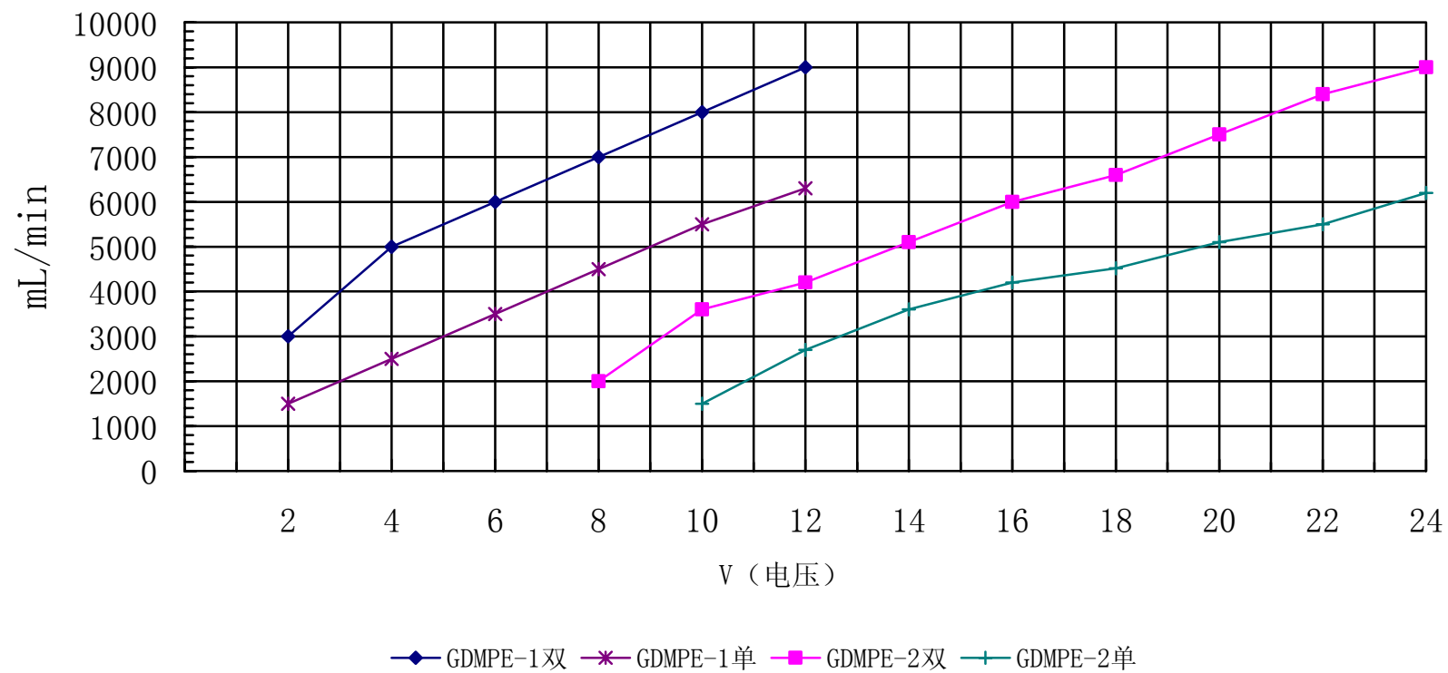
GDMPE电压流量图
