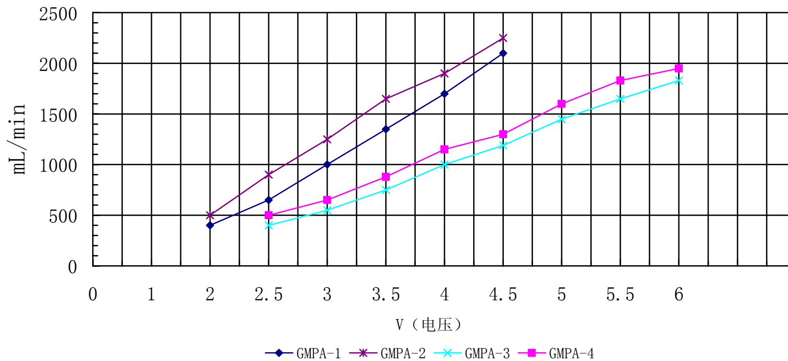
GMPA电压流量图
