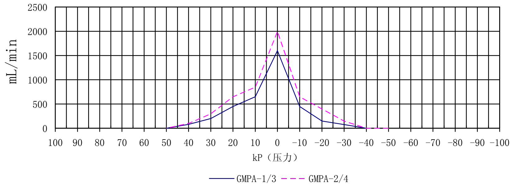
GMPA系列流量负载图
