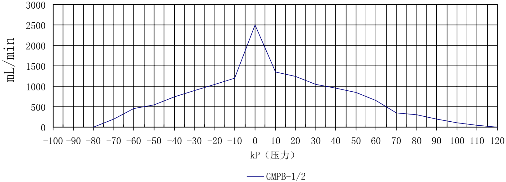
GMPB系列流量负载图
