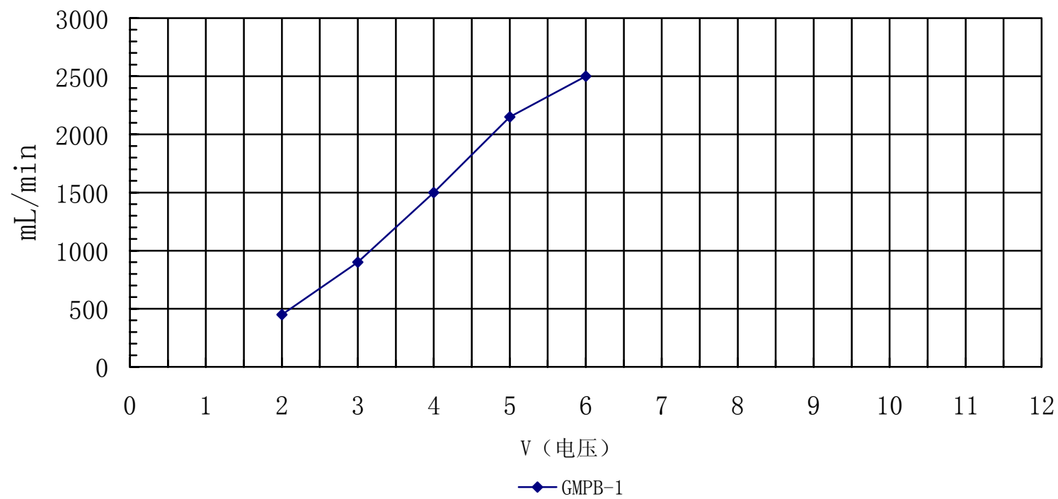
GMPB电压流量图
