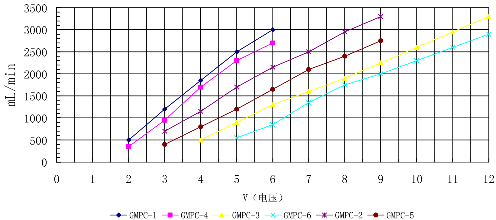
GMPC电压流量图
