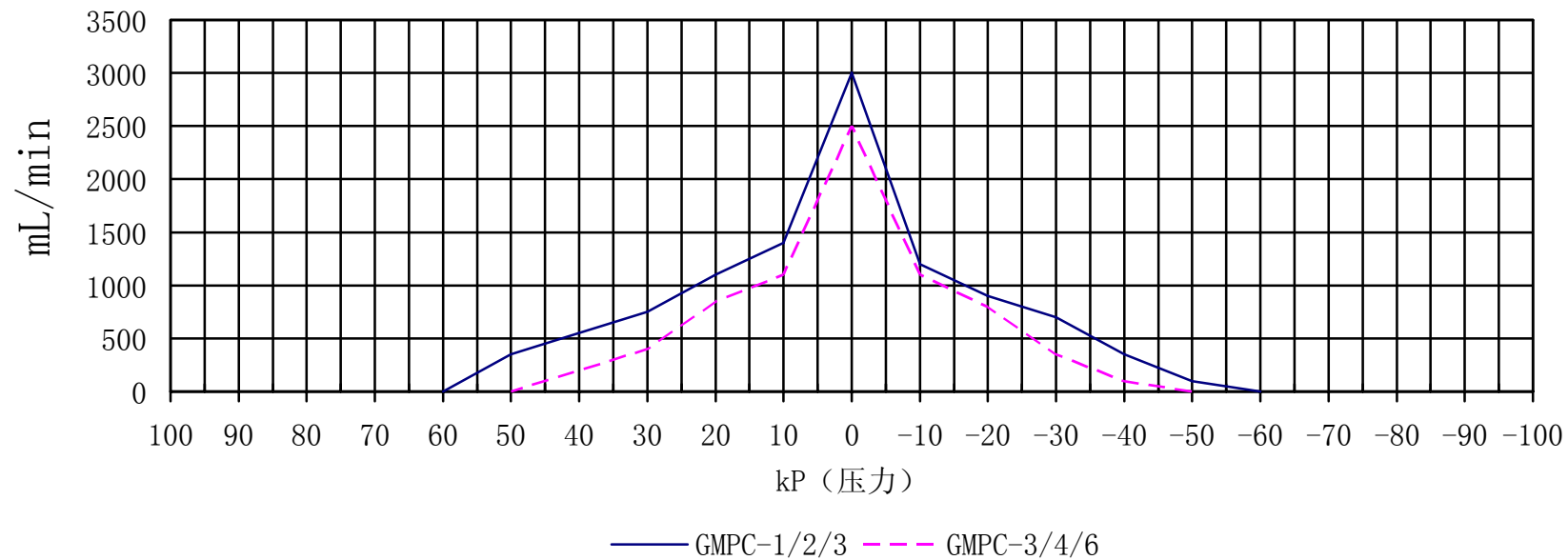
GMPC系列流量负载图
