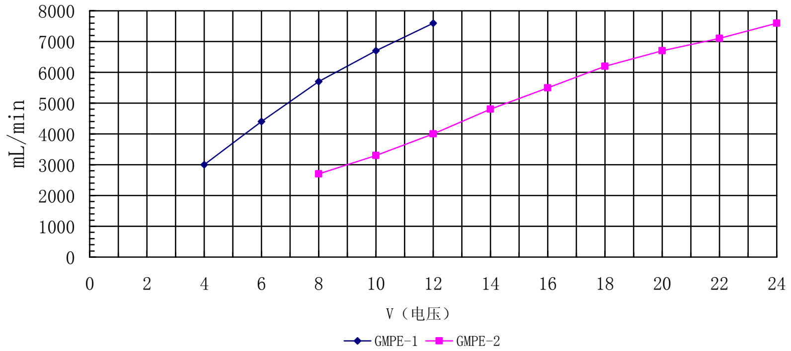
GMPE电压流量图
