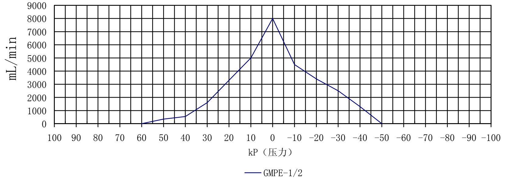
GMPE系列流量负载图
